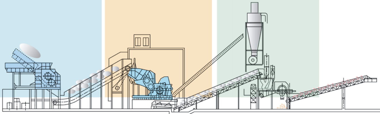
FNS-6080-1250 (1250馬カシュレディングプラント)
