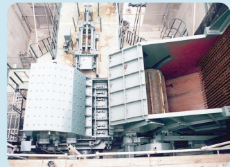
本体及び材料供給装置
